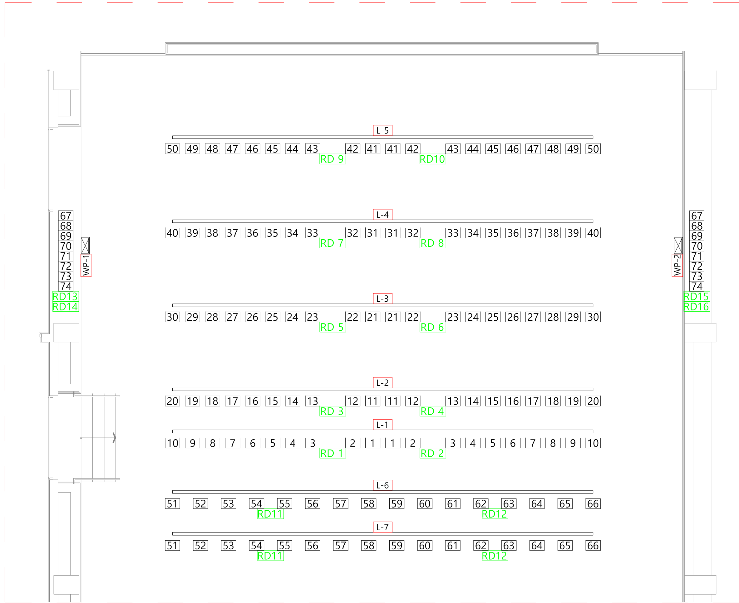
회로배치도 축척 : A3=1/60
